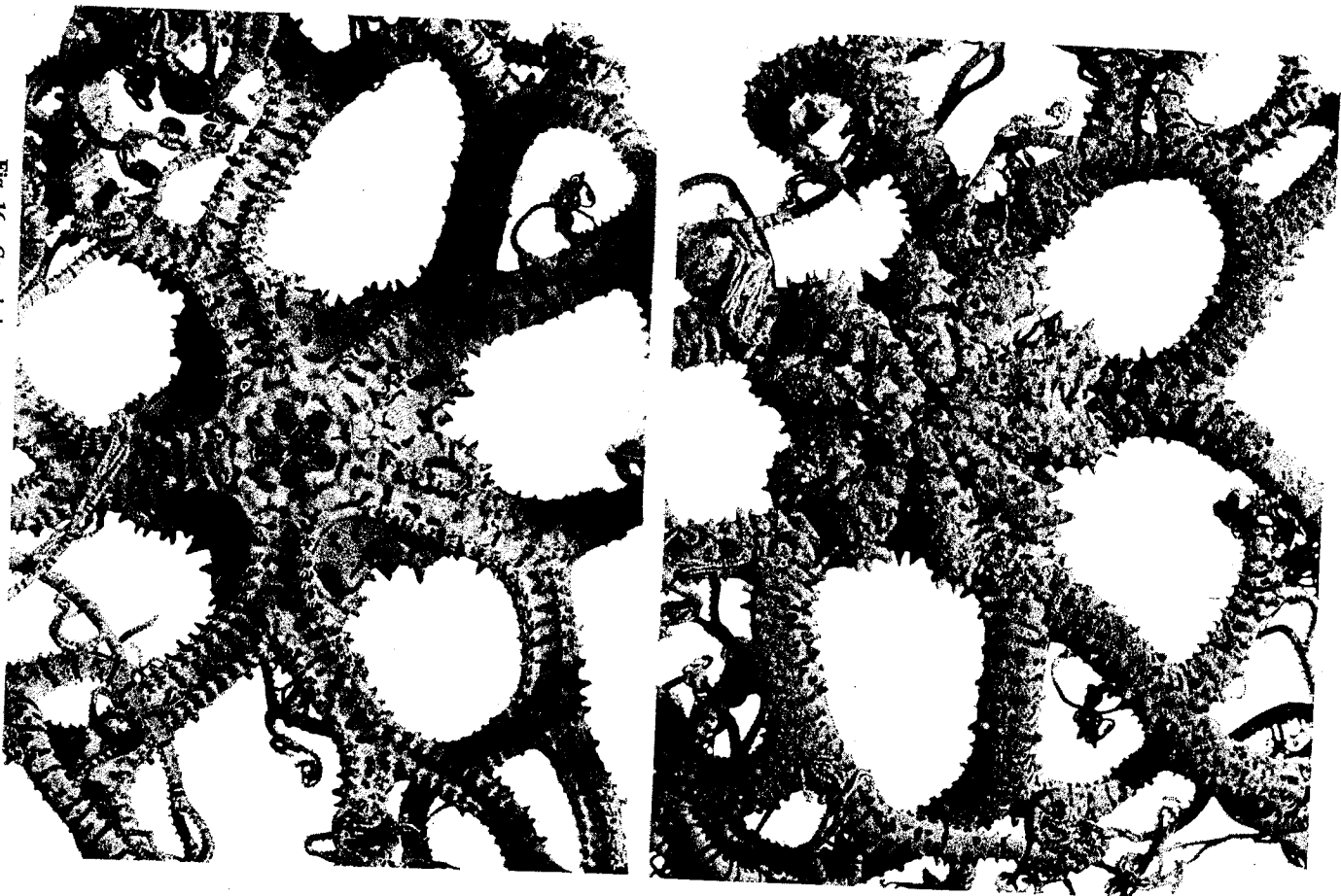
Fig. 16. Conocladus australis , Malacoota, Vic., 300 mm d.d.
