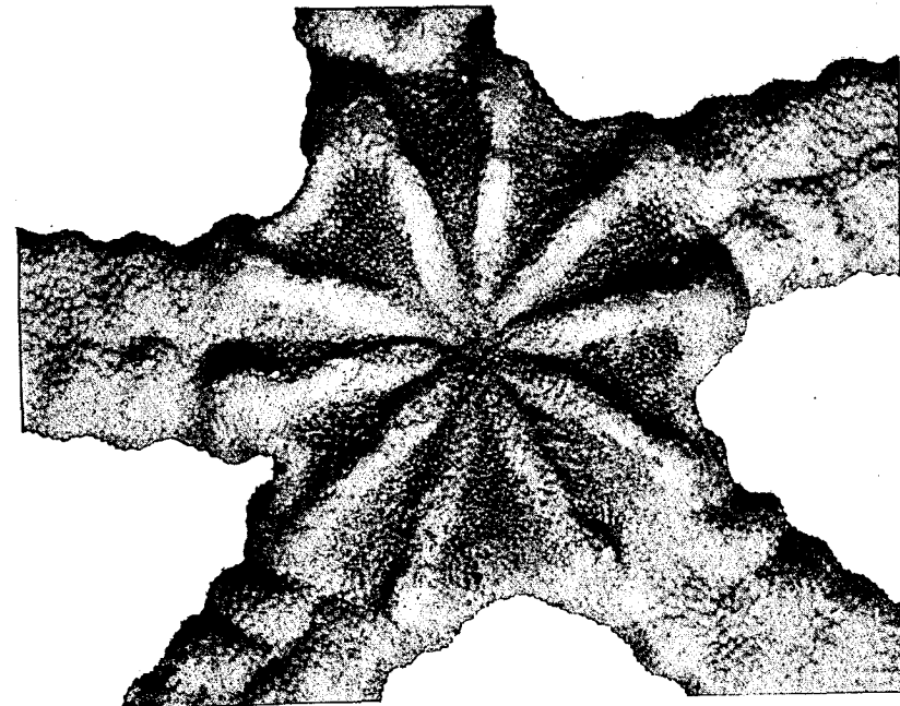
Fig. 4. Upper, Asteroschema horridum , Raoul I., 10.0 mm d.d.. Lower, A. tubiferum , Norfolk I., 14.0 mm d.d.
