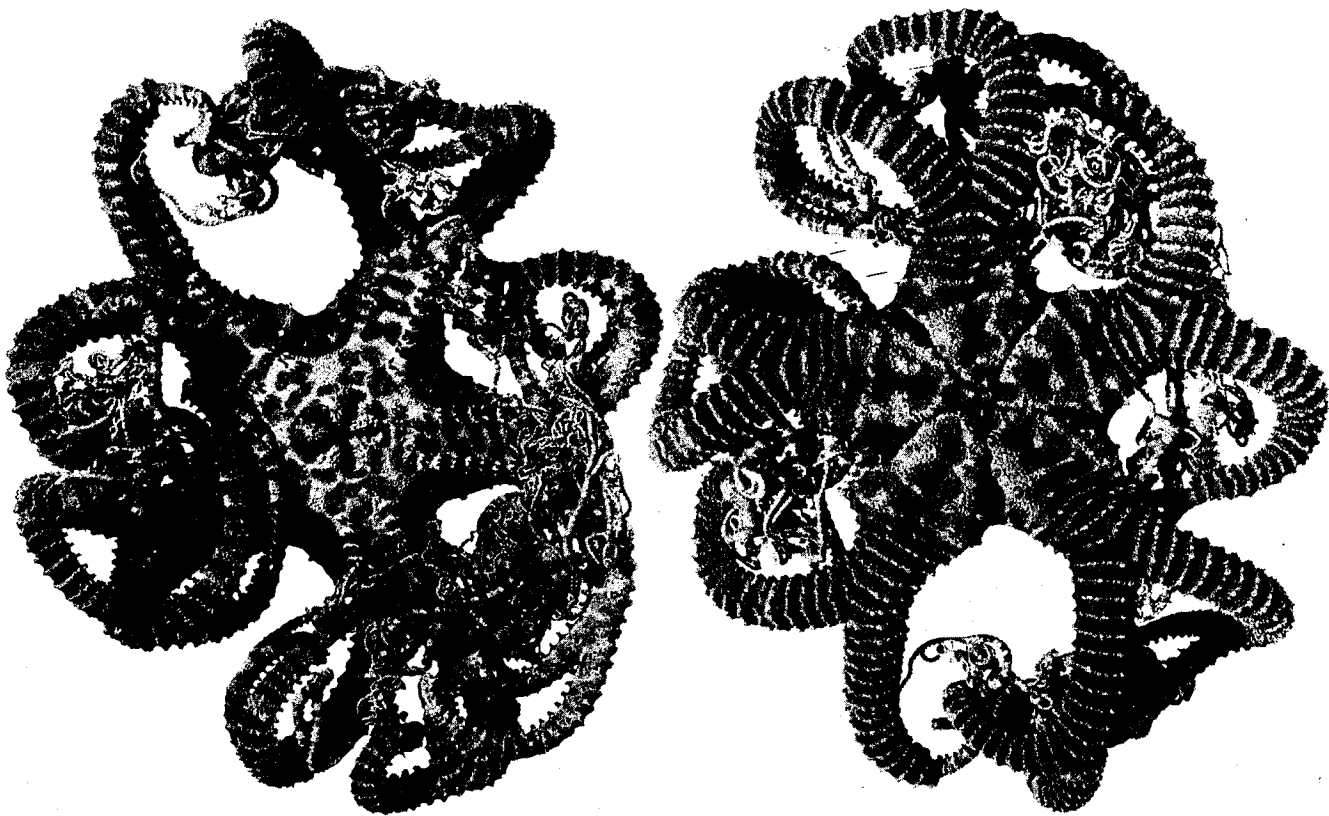
Fig. 17. Conocladus australis , Dunsborough, W.A., 260 mm d.d.
