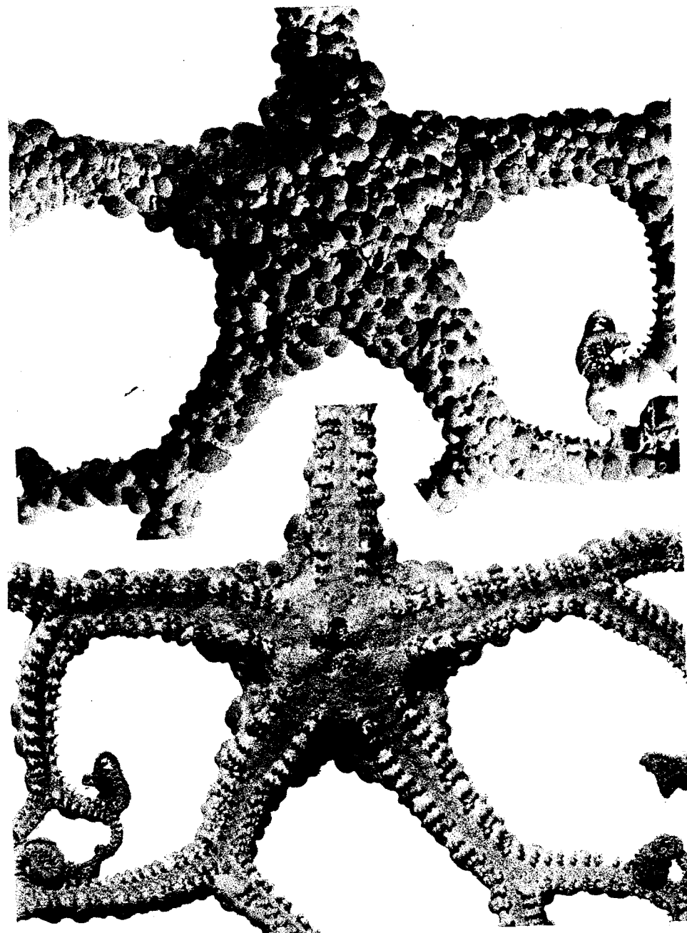
Fig. 13. Astrosierra amblyconus , Gabo I., Vic., 23.0 mm d.d.
