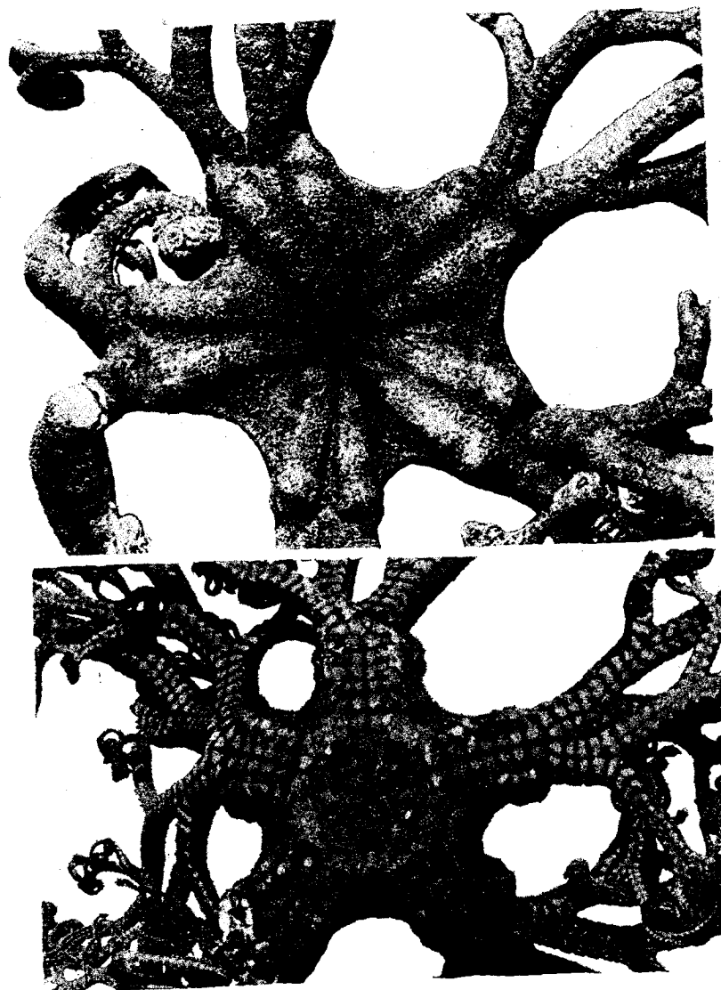
Fig. 24. Astrocladus tonganus , Tonga, 25.0 mm d.d.
